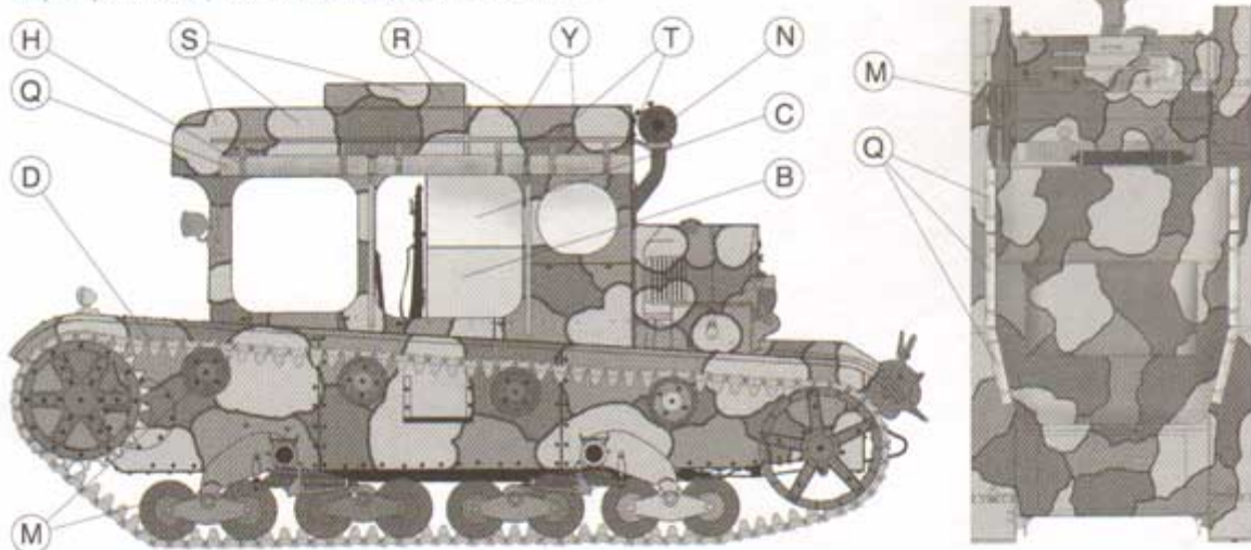
Ciężnik artyleryjski C7P Nr 8393 „FELEK” z BBT-Broni Panc. w trójbarwnym kamuflażu (tzw. japońskim). Rozkład plam patrz zdjęcia. Heavy artillery tractor C7P No 8393 „FELEK” from Armoured Weapon Techn. Research Bureau in three-tone camouflage („Japanese”). The camouflage scheme - see photos.
