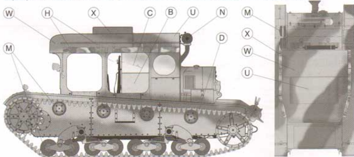
Ciężnik artyleryjski C7P „W0-597” z 2 Br Panc Żurawica w trójbarwnym kamuflażu (Polskim). Rozkład plam patrz zdjęcia. Heavy artillery tractor C7P „W0-597” from 2nd Armoured Brigade at Żurawica in three-tone camouflage (Polish). The scheme - see photos.
