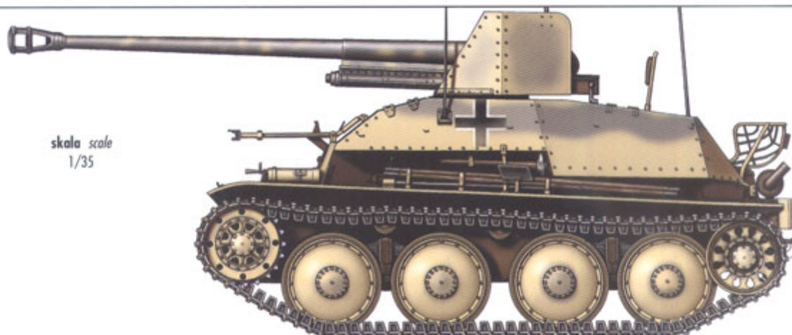
7,62 cm Pak (r) Fgst auf PzKpfw 38(t) [Sf] Sd Kfz 139 „Marder” III z 33. Zmot. Dywizjonu Niszczycieli Czołgów, Egipt, październik 1942 roku. 7.62cm Pak (r) Fgst auf PzKpfw 38(t) [Sf] Sd Kfz 139 "Marder" III SP gun of the 33rd Panzerjäger Abteilung (motorisiert), Egypt in October 1942.
