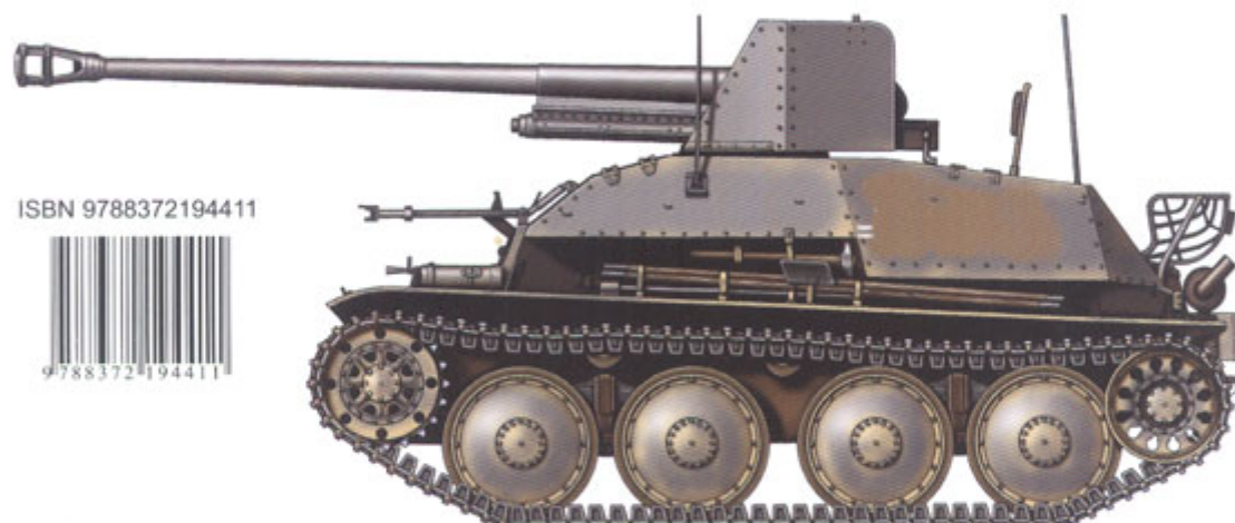
7,62 cm Pak (r) Fgst auf PzKpfw 38(t) [Sf] Sd Kfz 139 „Marder” III z 39. Zmot. Dywizjonu Niszczycieli Czołgów, Egipt, wrzesień 1942 roku. 7.62cm Pak (r) Fgst auf PzKpfw 38(t) [Sf] Sd Kfz 139 "Marder" III SP gun of the 39th Panzerjäger Abteilung (motorisiert), Egypt in September 1942.
